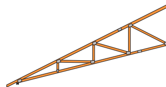
ハーフシザーストラス スパンの目安:~9.1m
